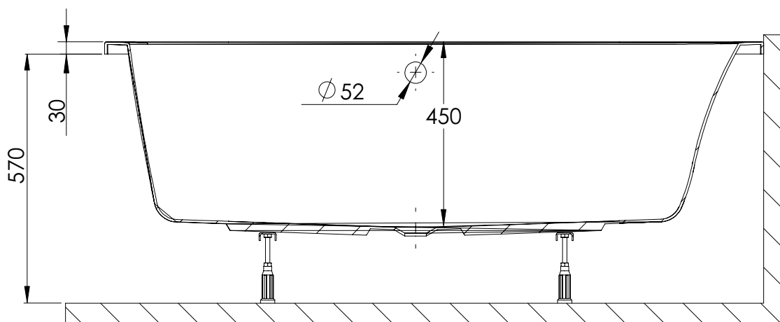
PRZEKRÓJ A-A
