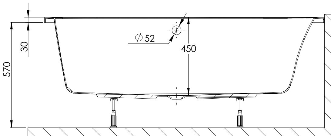
PRZEKRÓJ A-A
