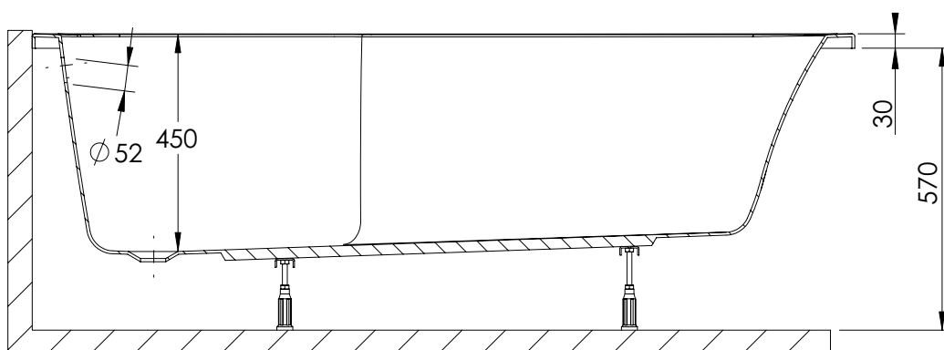
PRZEKRÓJ A-A
