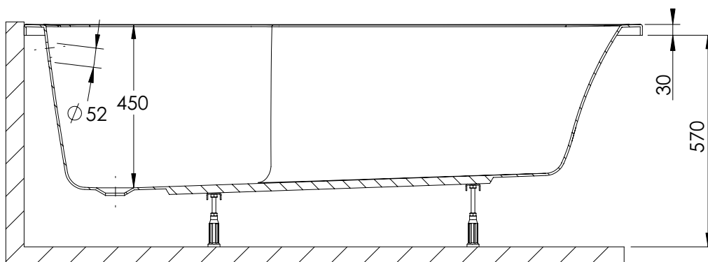
PRZEKRÓJ A-A
