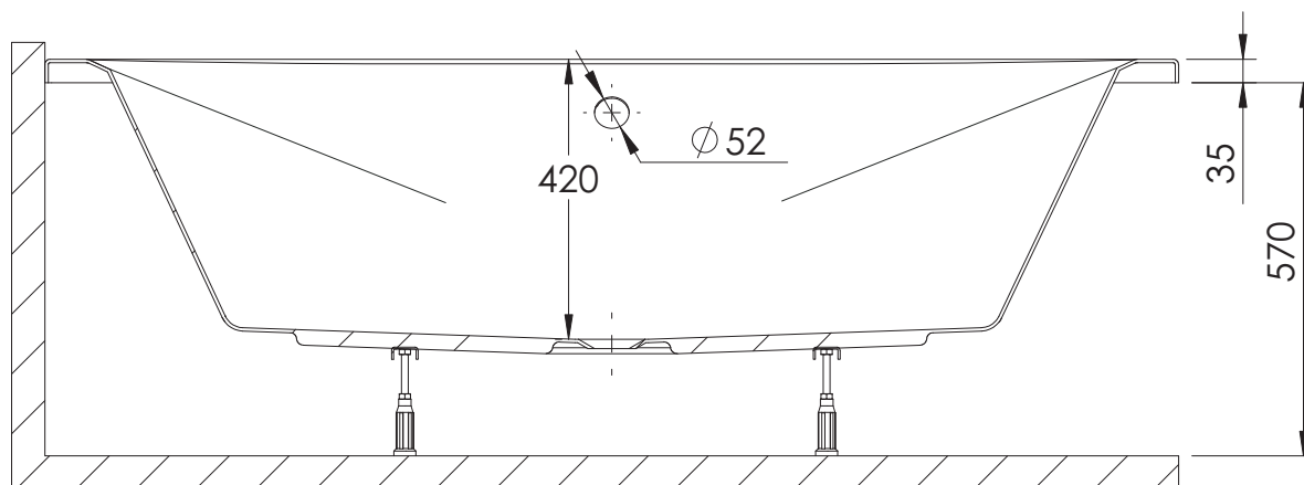
PRZEKRÓJ A-A
