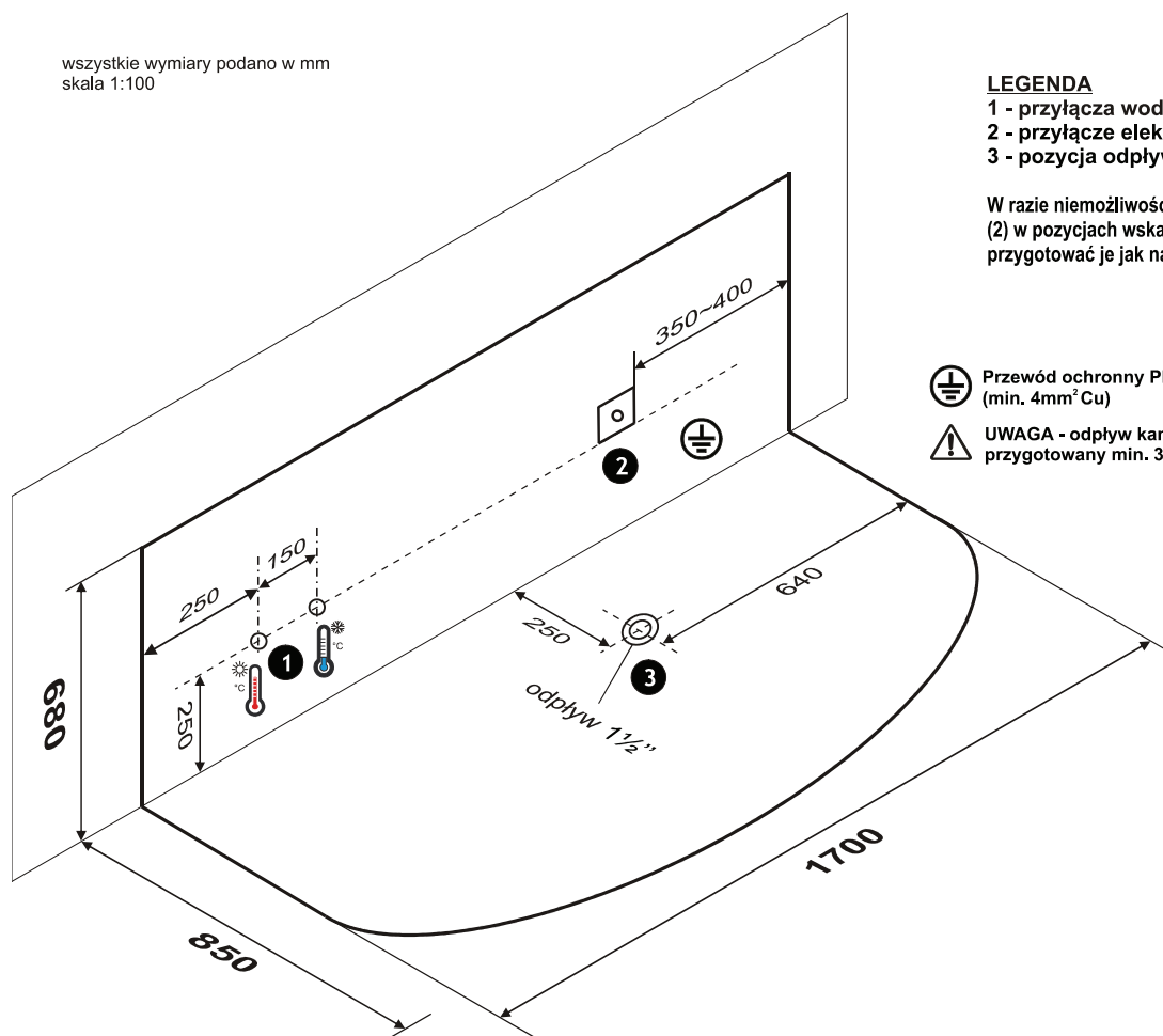
rys. 4 - zalecane miejsca przygotowania przyłączy
