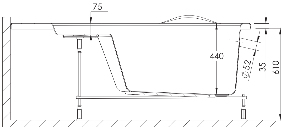
PRZEKRÓJ A-A
