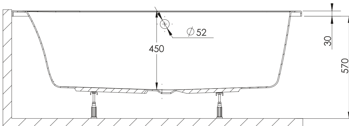
PRZEKRÓJ A-A
