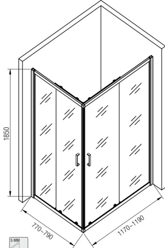
KABINA PRYSZNICOWA MEXO 800x1200x1850 (nr art. VL.A1800F.80.120)
