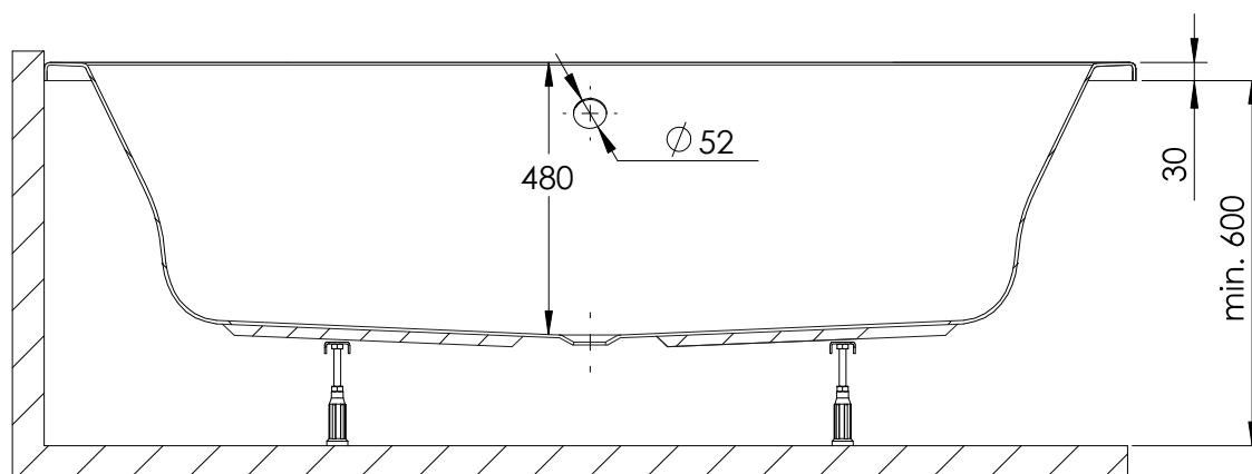
PRZEKRÓJ A-A
